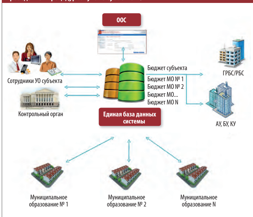
Рисунок 1. Централизованное решение при автоматизации управления проведением процедур закупок в субъекте РФ
