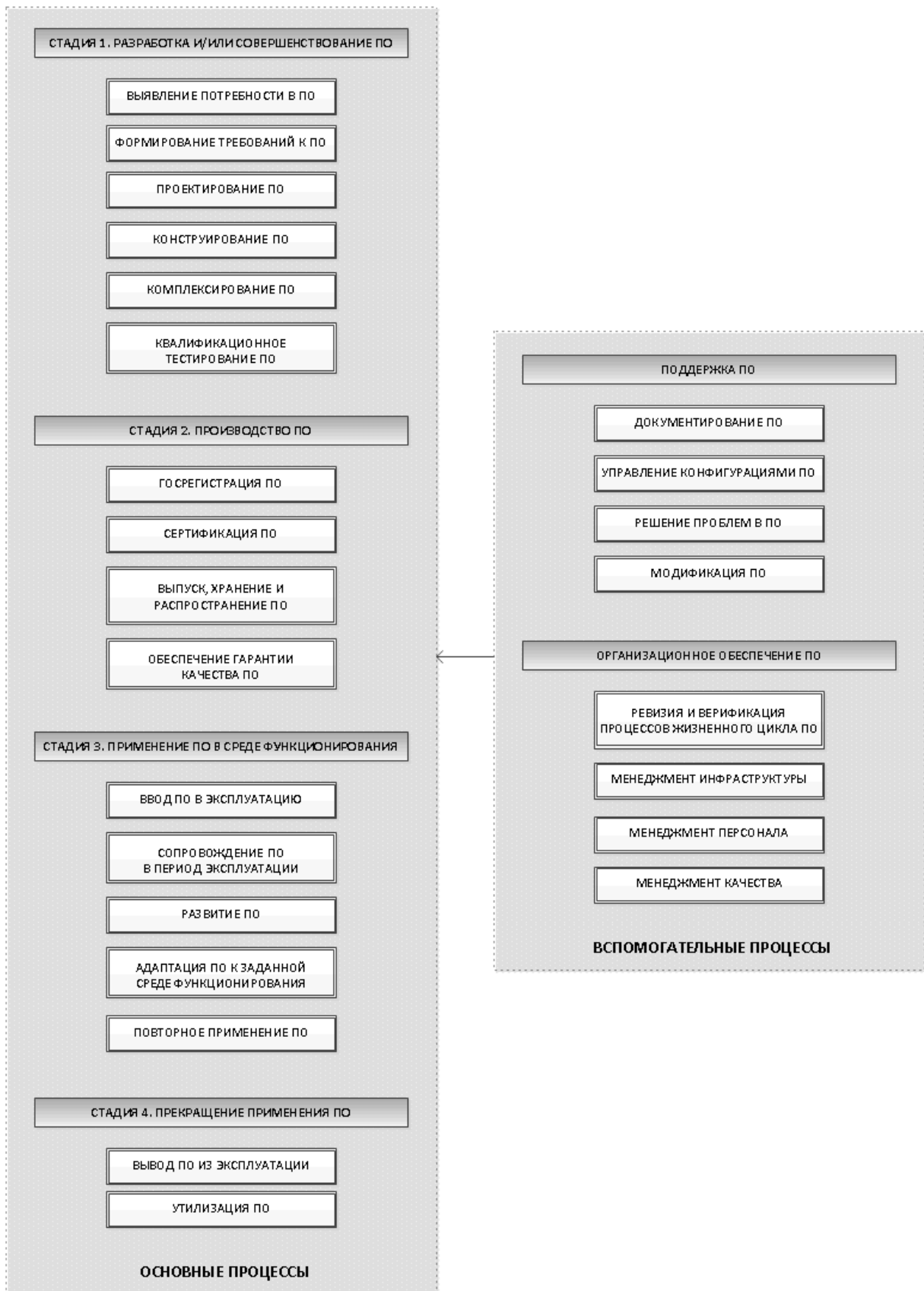
Рисунок 1. Модель жизненного цикла ПО для Системы
