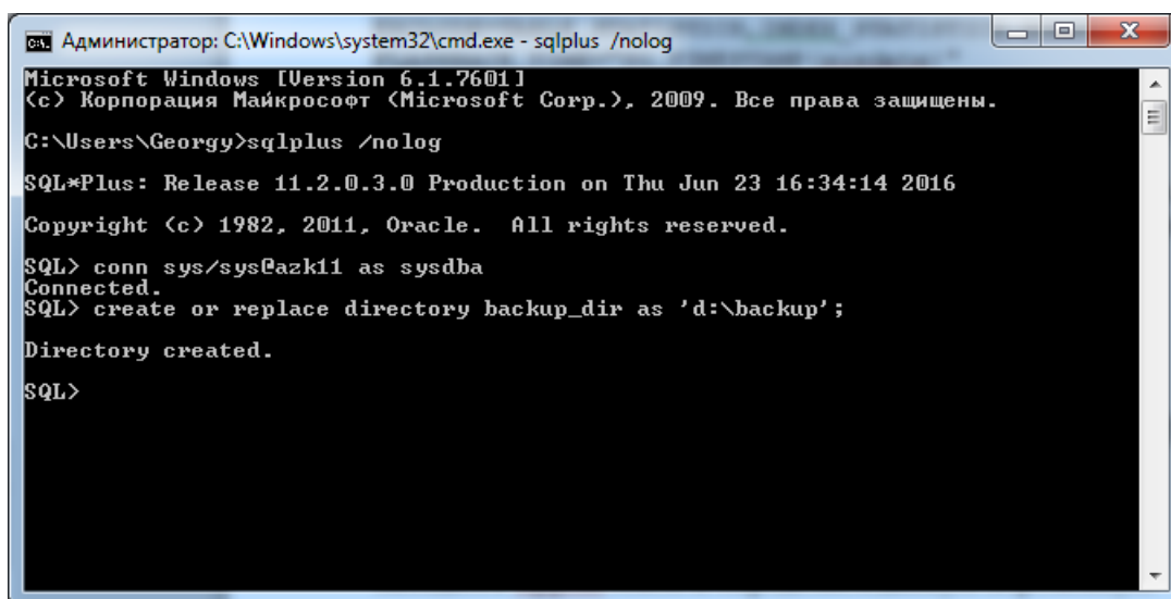
Рисунок 33 – Определение переменной backup_dir
