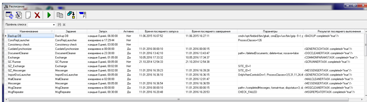
Рисунок 30 – Расписание планировщика
