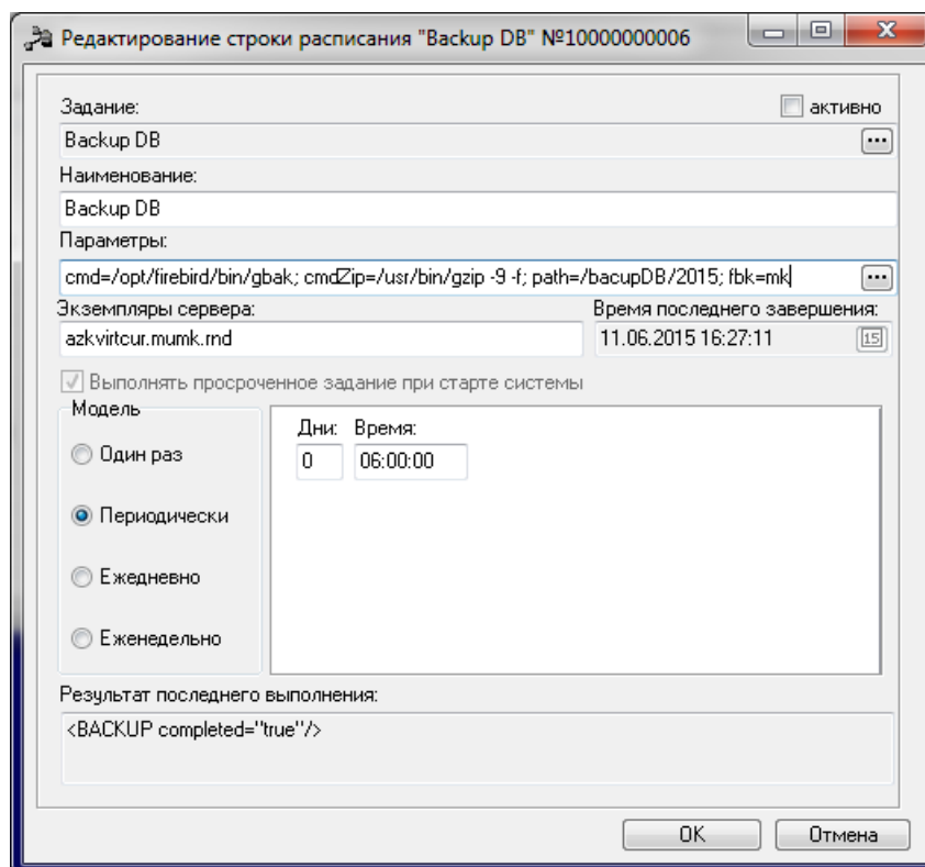
Рисунок 32 – Форма редактирования строки расписания
