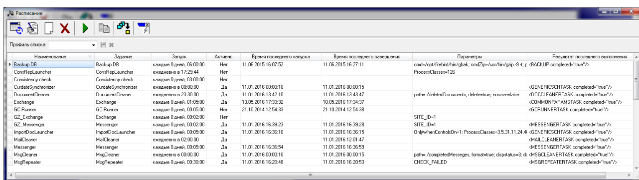
Рисунок 31 – Расписание планировщика
